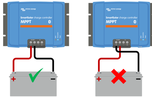
Ejemplos de polaridad de la batería correcta e incorrecta (invertida)
