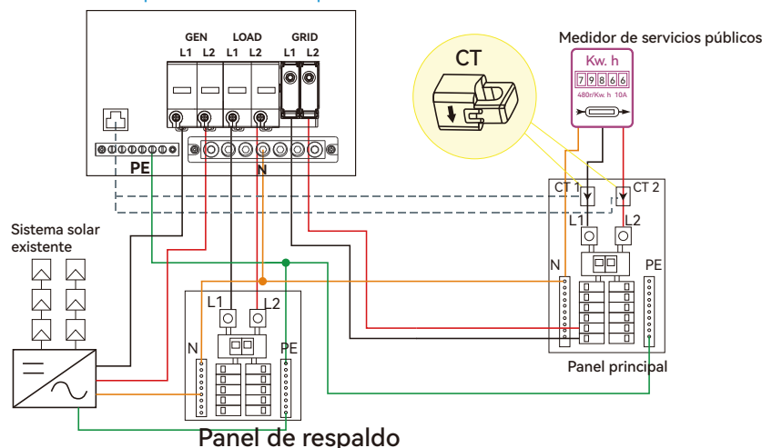
Conexión para sistema solar acoplado a CA
