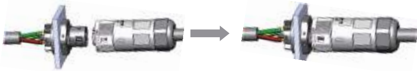
Figura 4.18 Cómo conectar el conector de CA al inversor
