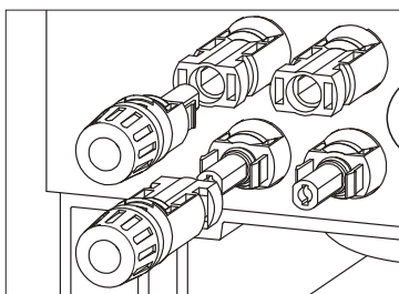
Figura 4.12 Conexión al inversor
