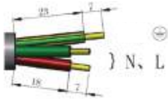
Figura 4.15 Cables de CA pelados
