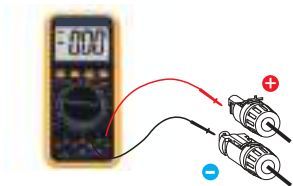
Figura 4.11 Medición con multímetro
