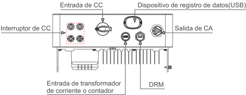
Figura 1.2 Vista inferior
