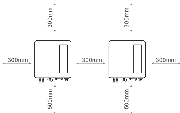
Figura 4.2 Distancia de montaje del inversor
