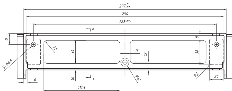
Figura 4.3 Montaje del inversor en la pared
